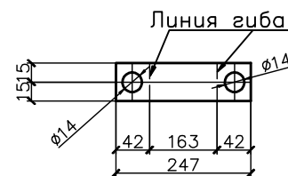
Развертка поз.5
