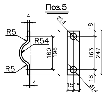
Развертка поз.5
